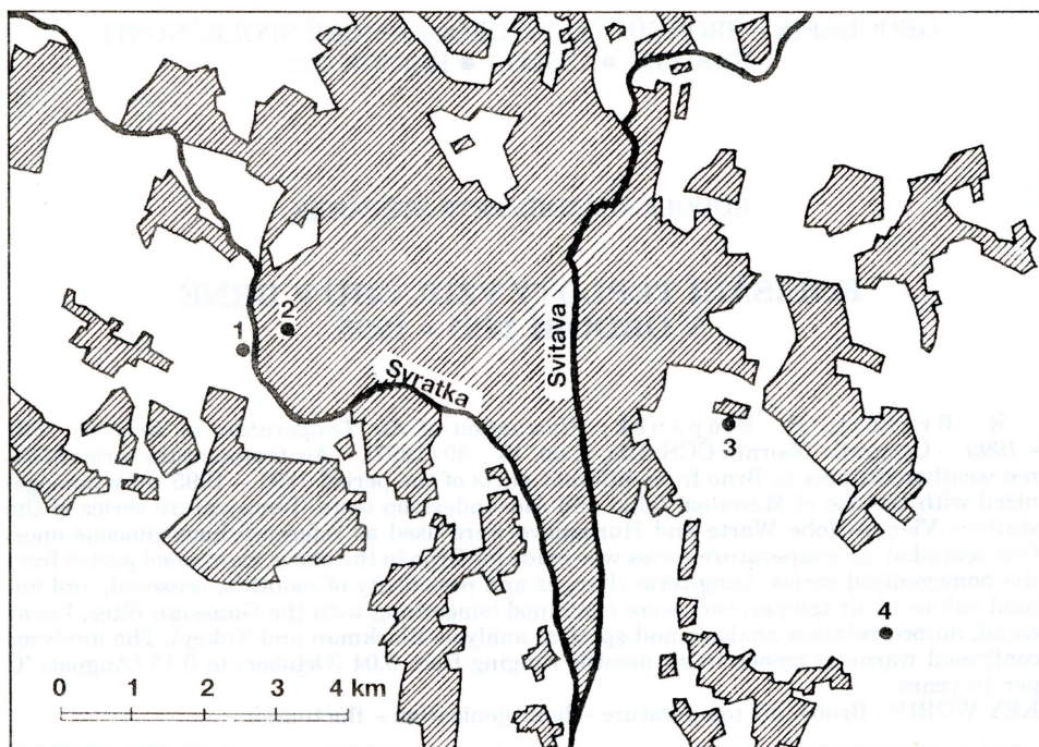
Obr. 1 – Schematická mapka Brna s vyznačením polohy použitých meteorologických stanic: 1 – Brno-Pisárky, 2 – Brno-Květná, 3 – Brno-letišťe (před rokem 1958), 4 – Brno-letišťe (od roku 1958). Šrafovaně je vyznačena souvisle zastavěná plocha.
